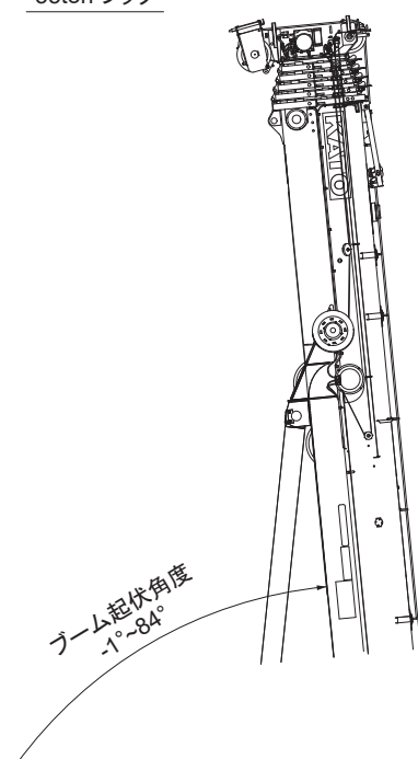
55ton フック
