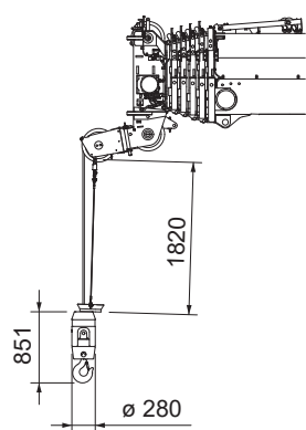
5.6ton フック
