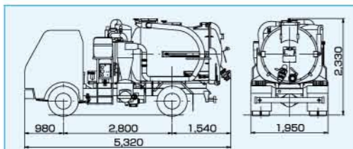
MV-400Sリフトアップ仕様
