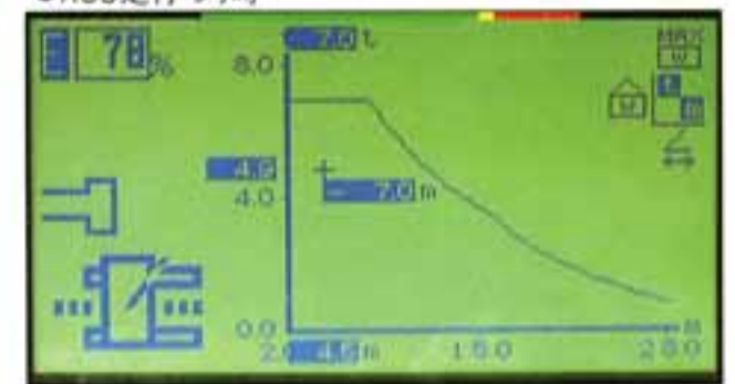
●作業半径性能カーブ時
