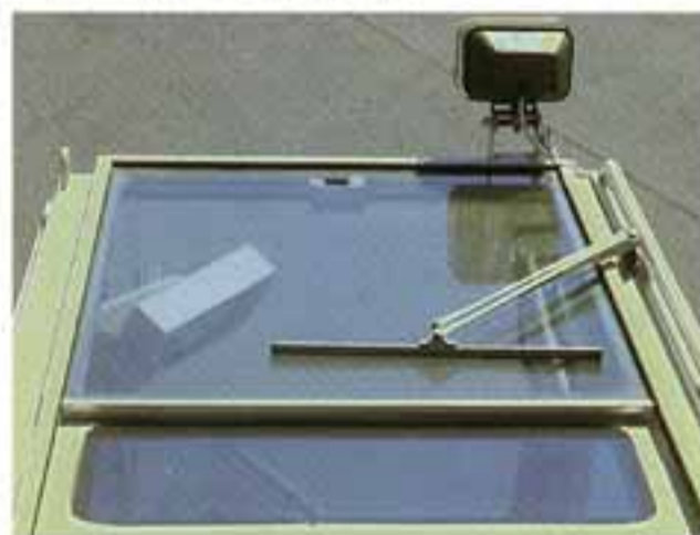
● ワイパー付のスライド式大型ルーフウィンドを採用
