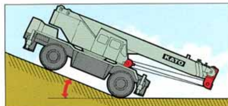
●アプローチアングル(進入角)
